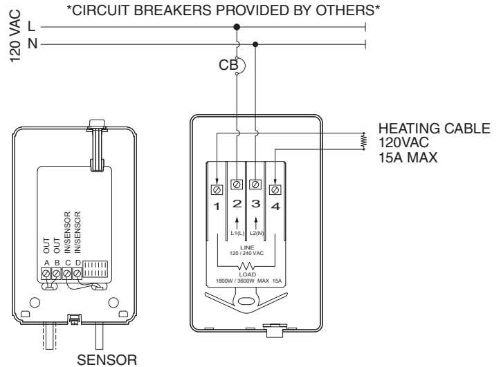
Detail 2. UDG-4999 120 VAC wiring diagram.
