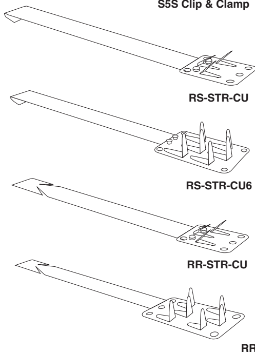
S5S Clip & Clamp
